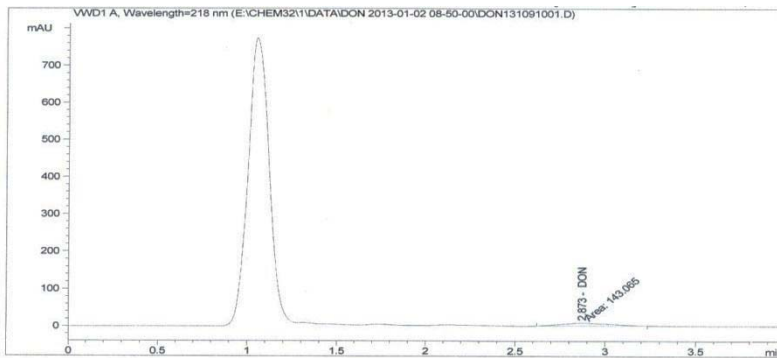
نمودار ۴: کروماتوگرام HPLC و منحنی استاندارد برای محاسبه غلظت داکسی نیوالنول در نمونه های برنج
