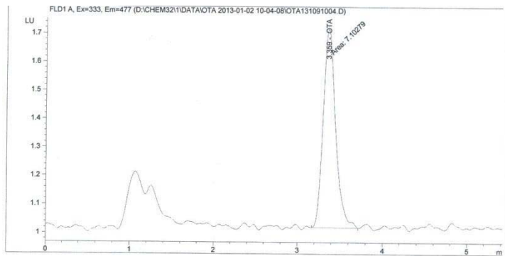
نمودار ۲: کروماتوگرام HPLC و منحنی استاندارد برای محاسبه غلظت اکراتوکسین در نمونه های برنج
