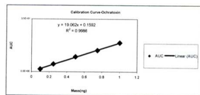
نمودار ۲: کروماتوگرام HPLC و منحنی استاندارد برای محاسبه غلظت اکراتوکسین در نمونه های برنج
